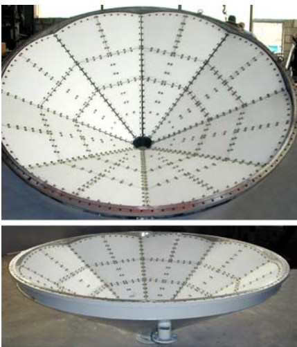
Homogenisierboden
