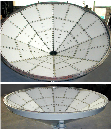
Homogenisierboden
